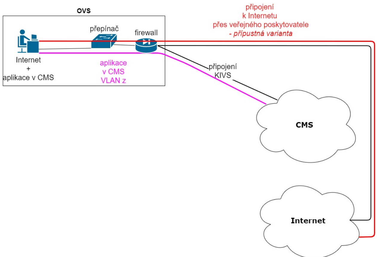
Obrázek 5: Příklad připojení OVS ke službám CMS přes KIVS, kdy provoz uživatele je virtuálně oddělen od ostatního provozu – tento uživatel má zároveň přístup i k Internetu – přípustná varianta připojení k Internetu
